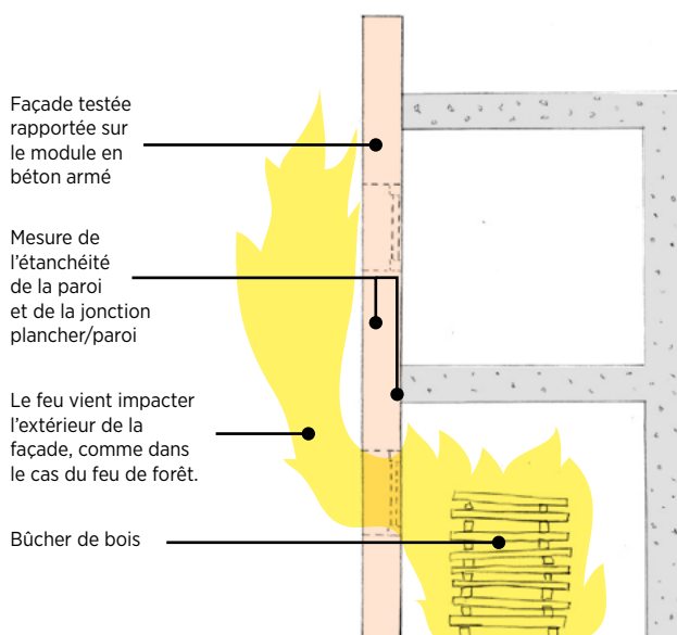
Essai au feu LEPIR 2. Les flammes sont produites par la combustion du bûcher, non par celle des matériaux de construction.
