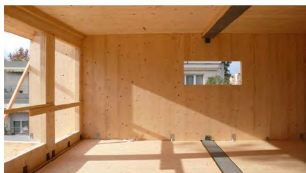
Construction en CLT en cours de montage
