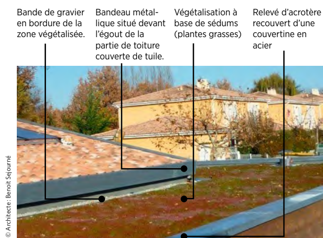
Exemple de toiture terrasse végétalisée
